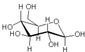
Glucose (Hemiacetal)
